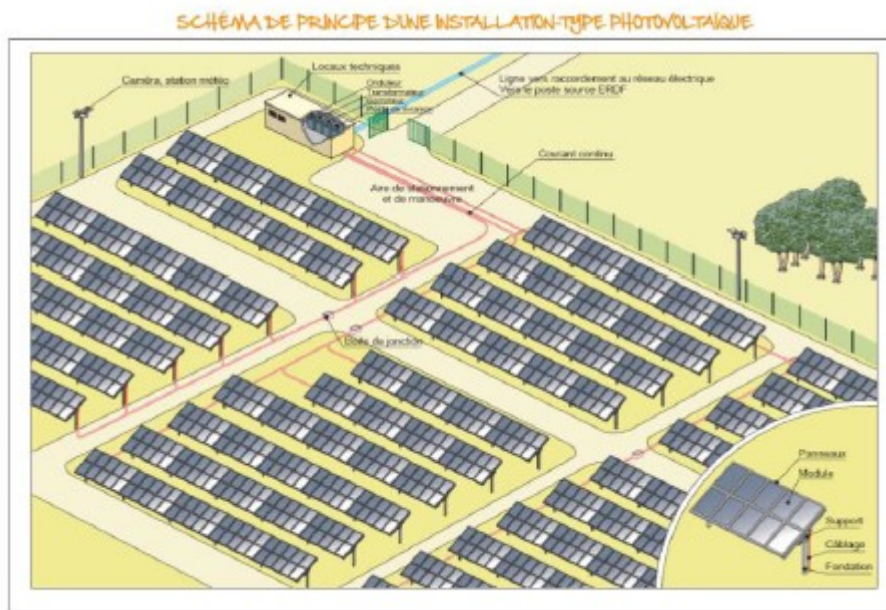
Illustration 2: Schéma de principe du projet (source : étude d'impact – figure 17 p.52)
