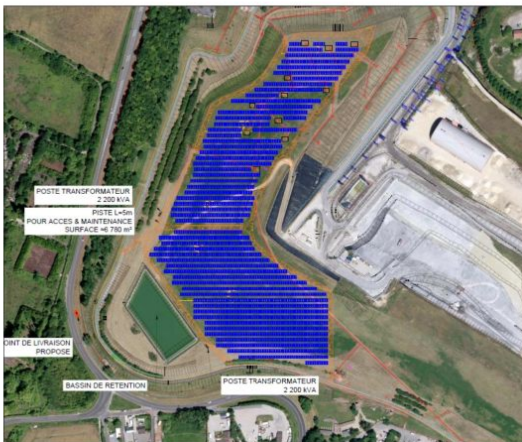
Figure 4 : Plan du projet - Source : étude d'impact (p 38)
