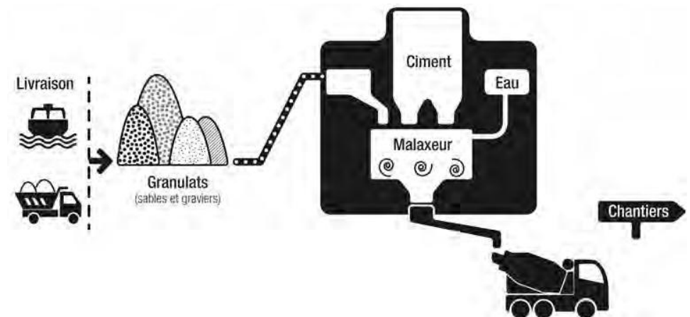
Figure 18 : Schéma explicatif du fonctionnement d'une centrale à béton (source : panorama des granulats en Île-de-France, 2017).
