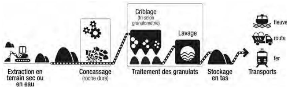
Figure 16 : Fonctionnement d'une carrière de granulat (source : panorama des granulats en Île-de-France, 2017).
