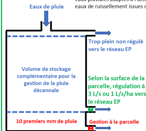
Figure 2.1 : Logigramme de gestion des eaux pluviales
