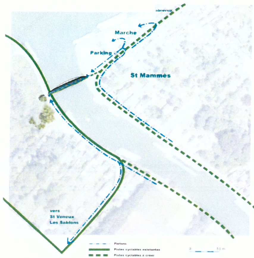
Positionnement de l'ouvrage à la confluence Loing-Seine
