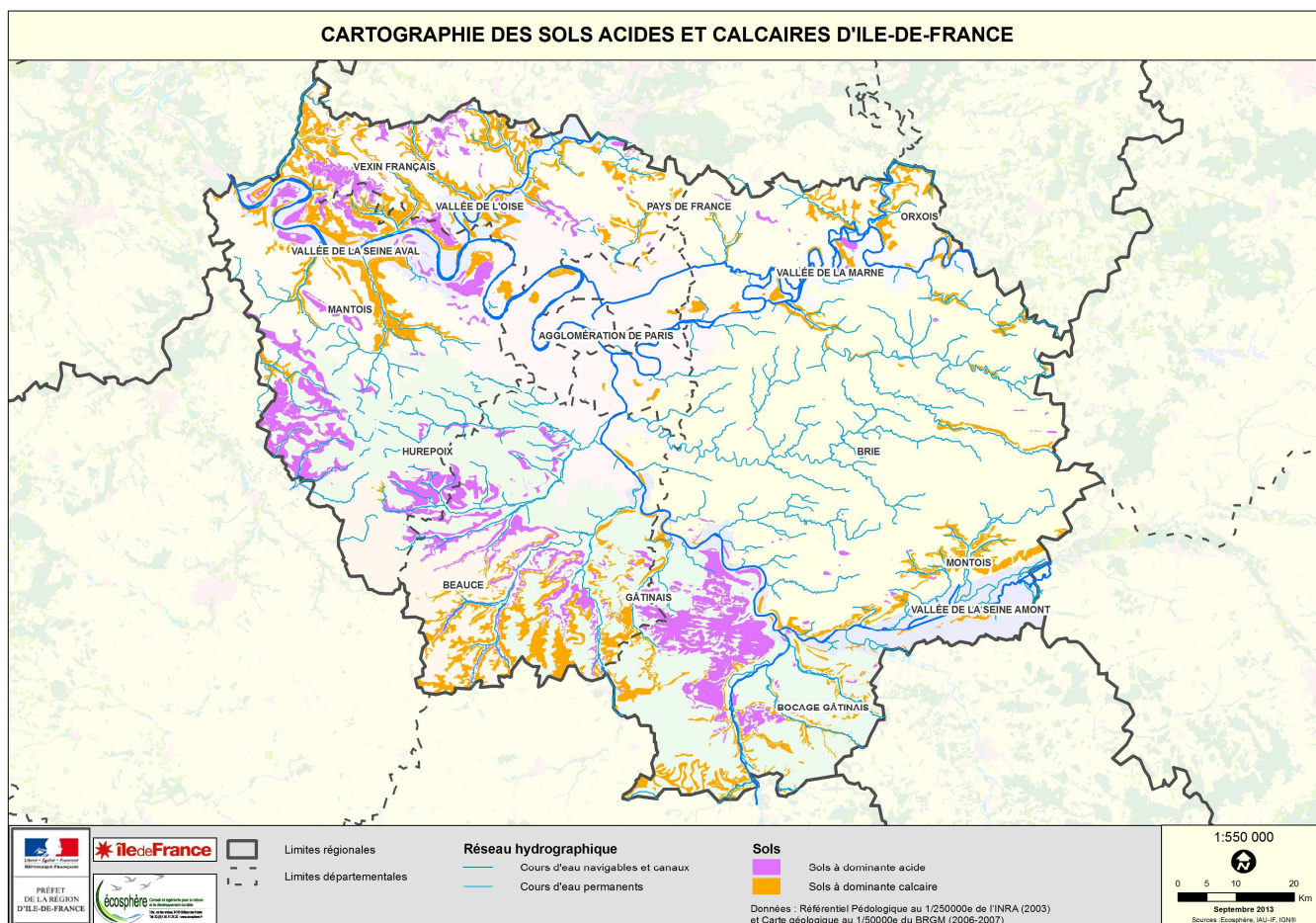
Carte 2. Cartographie des sols acides et calcaires d'Île-de-France
