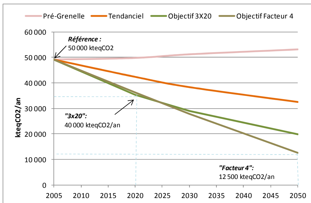
Graphique 4. Scénarios d'évolution des émissions de gaz à effet de serre (Source : SRCAE Île-de-France V1)
