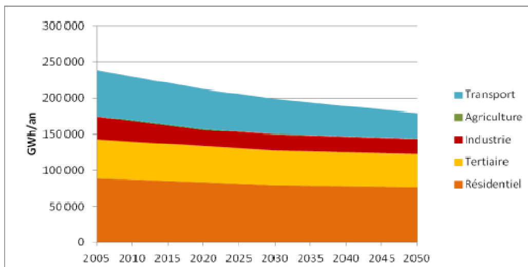
Graphique 3. Evolution tendancielle des consommations énergétiques par secteur (Source : SRCAE Île-de-France V1)
