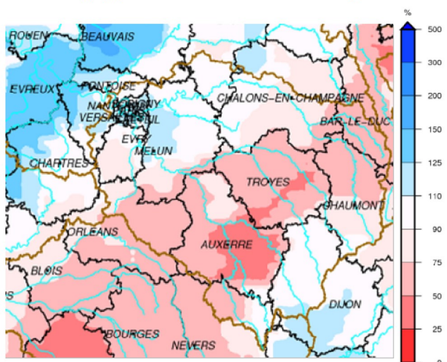
Carte de la pluie du mois d'octobre 2021 (rapportée à la normale 1981-2010)
