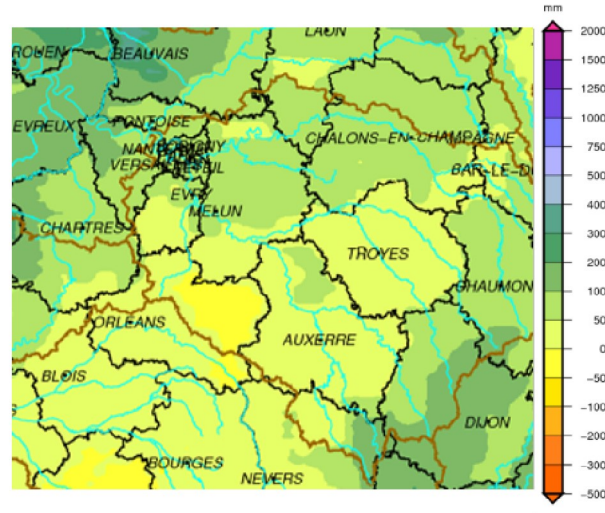
Carte de la pluie efficace du mois d'octobre 2021 (pluie efficace = pluie - évapotranspiration)
