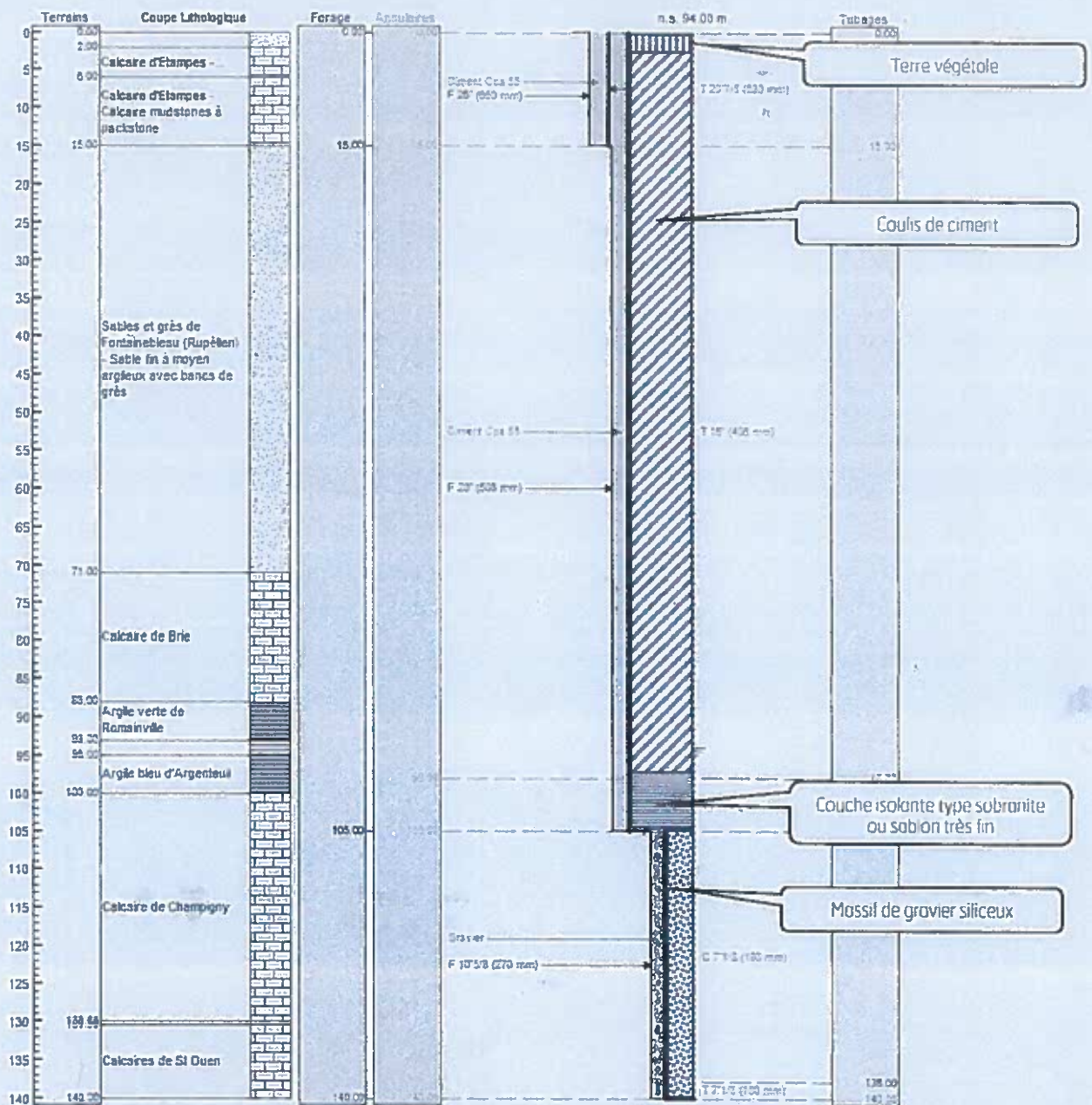
Figure 8 : coupes technique et lithostratigraphique du forage comblé prévisionnelles (12/12/2018)
