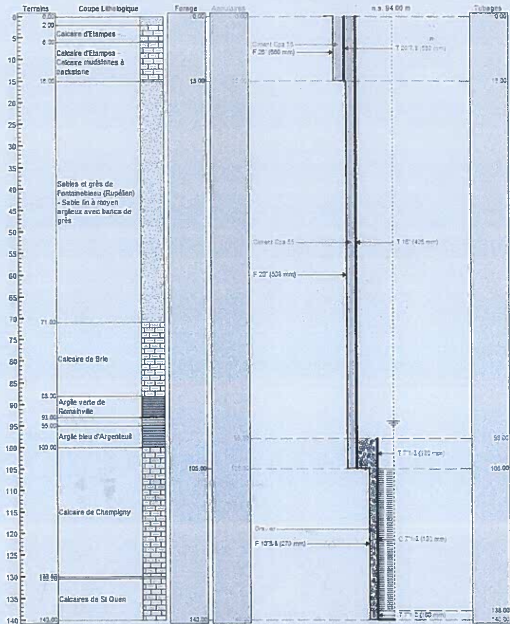
Figure 7 : coupes technique et lithostratigraphique du forage prévisionnelles (12/12/2018)
