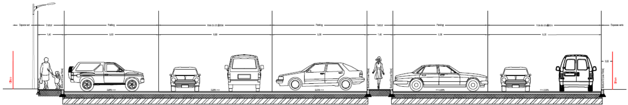
Figure 11 : Coupe de principe
