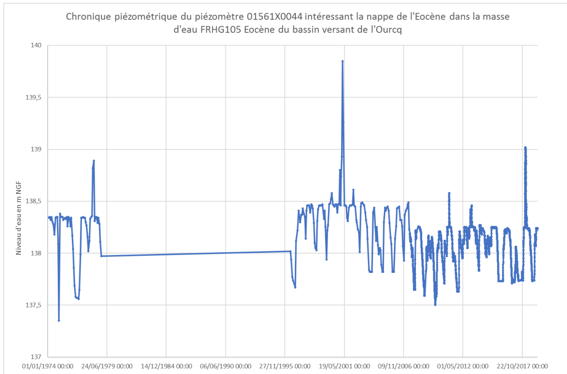
Chronique piézométrique de la nappe de l'éocène de 1969 à 2019
