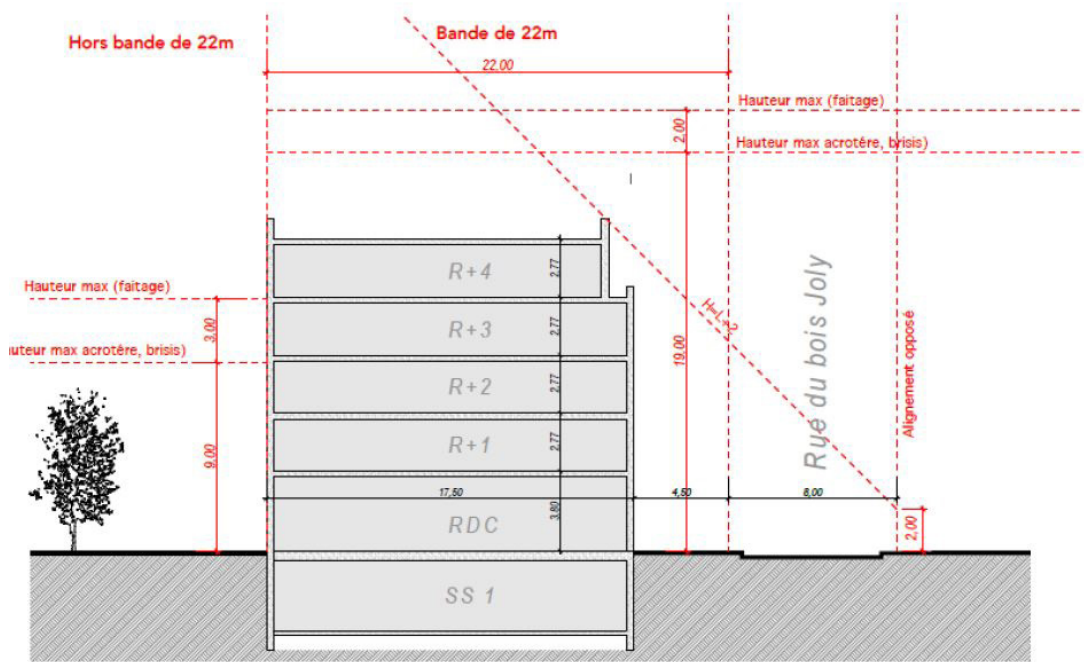
Coupe BB
