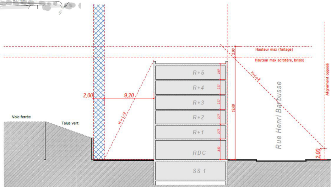
Coupe AA
