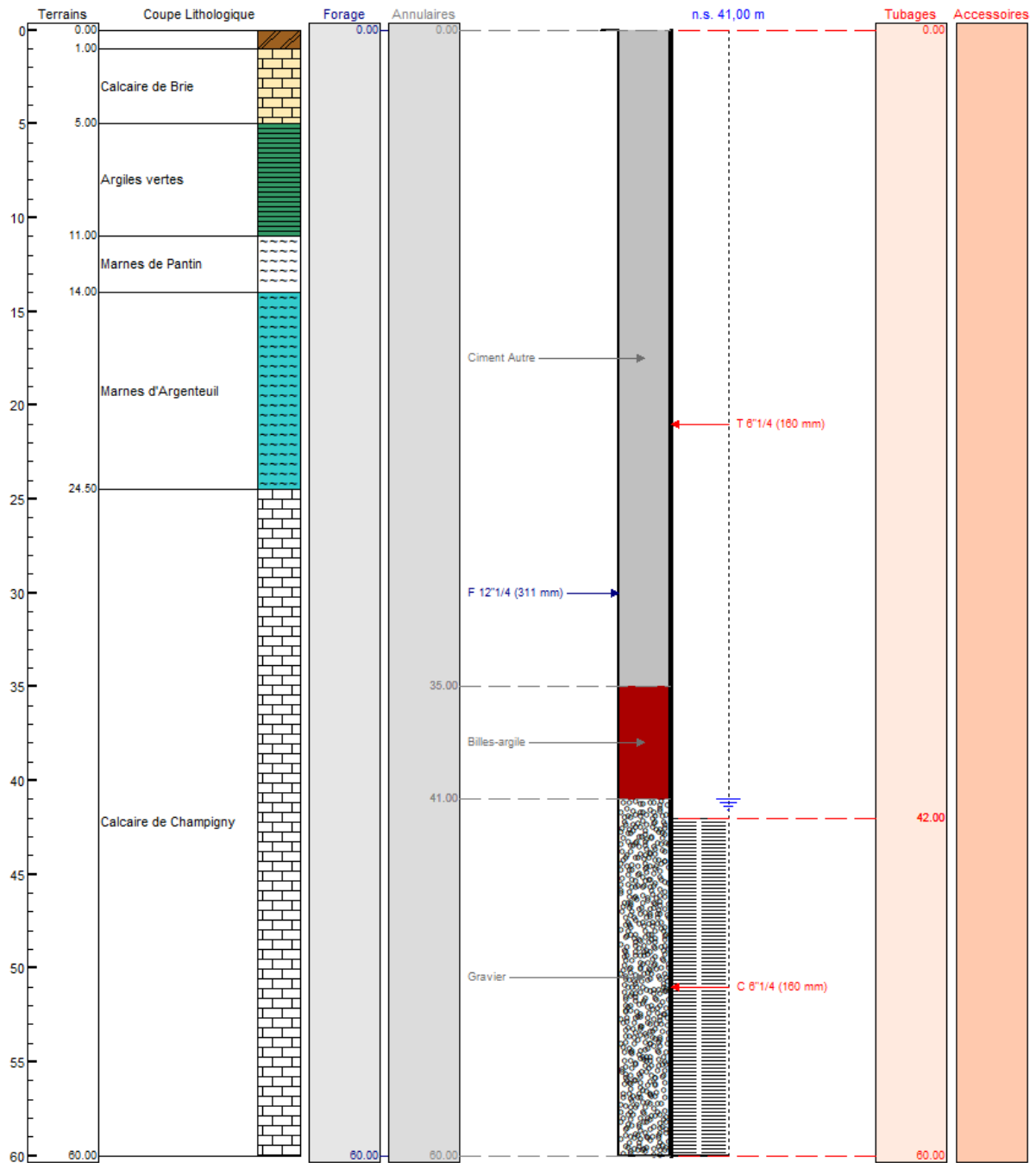
Coupe technique et géologique prévisionnelle du forage au Champigny
