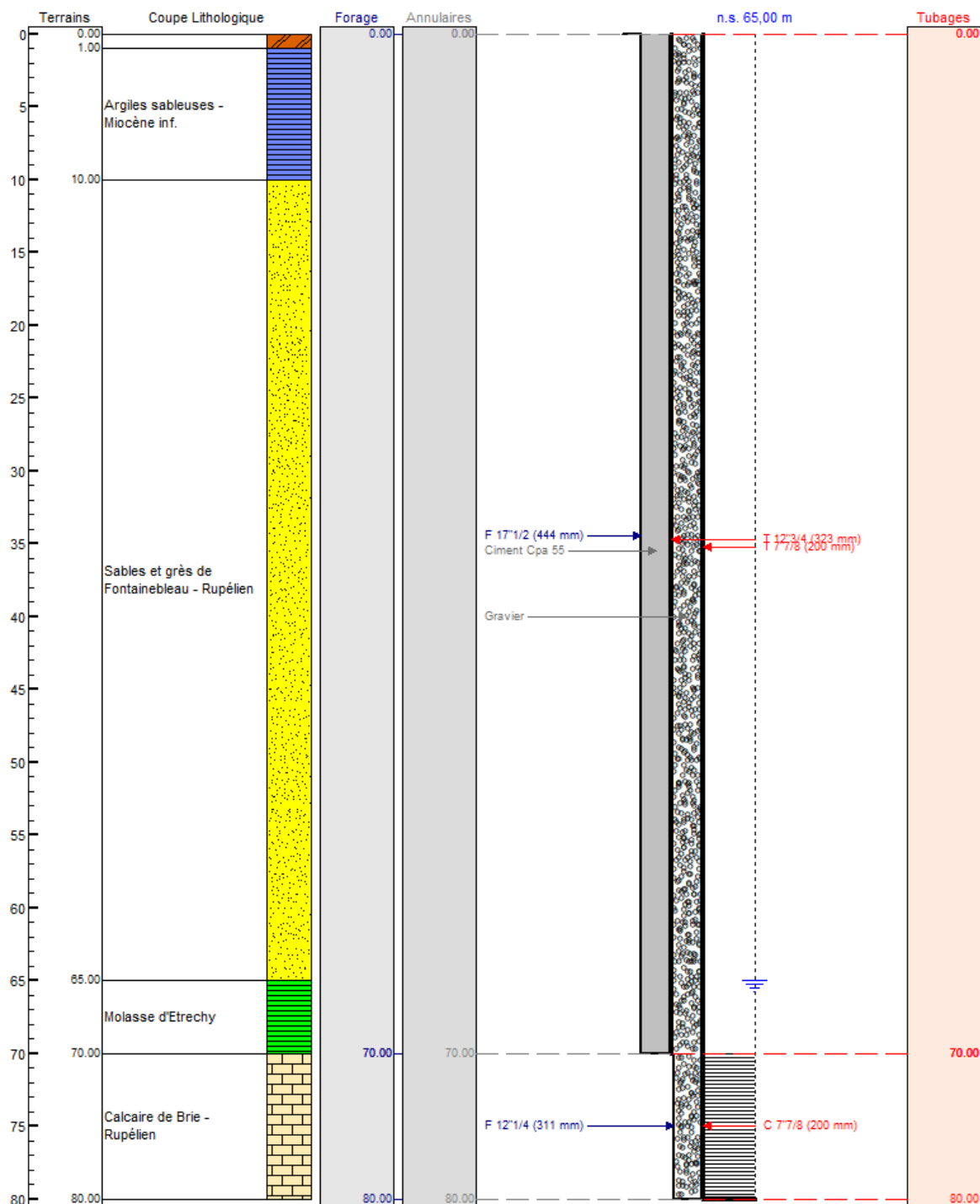
Figure 12 : coupes technique et géologique prévisionnelles des forage F1 et F2
