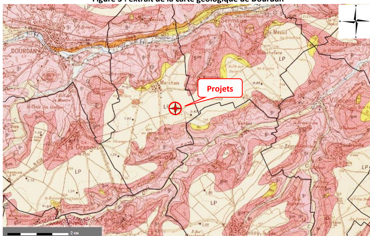
Figure 3 : extrait de la carte géologique de Dourdan
