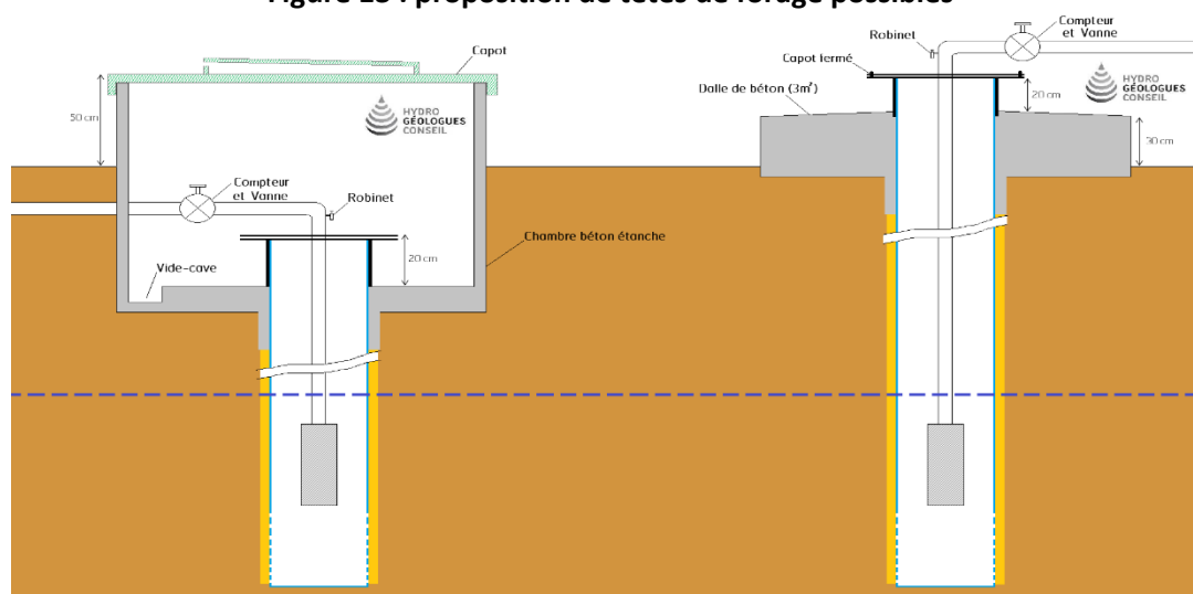
Figure 13 : proposition de têtes de forage possibles
