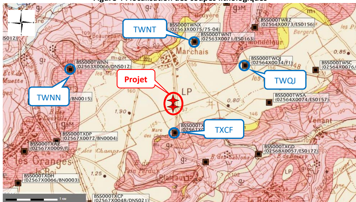
Figure 4 : localisation des coupes lithologiques
