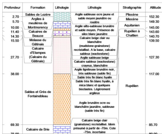
Figure 6 : géologie au droit de l'ouvrage BSS000TWNN (TN = + 155 mNGF)
