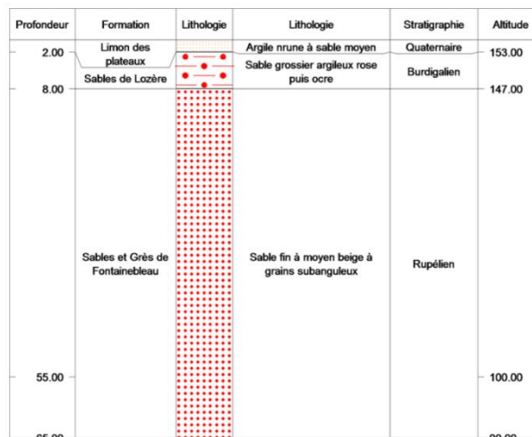
Figure 7 : géologie au droit de l'ouvrage BSS000TWNT (TN = + 155 mNGF)
