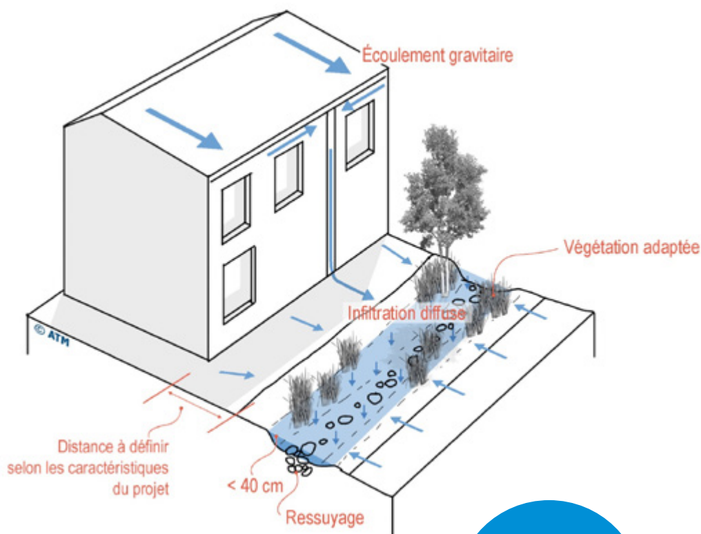
AXONOMETRIE JARDIN DE PLUIE EN PIED DE BATIMENT
