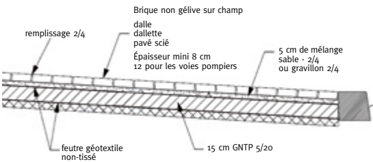
COUPE TYPE D'UNE STRUCTURE RESERVOIR SOUS TROTTOIR AVEC REVETEMENT PERMEABLE.
