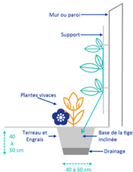
SCHEMA TYPE DE MISE EN PLACE D'UNE VÉGÉTALISATION DE FAÇADE EN PIED DE MUR Source : STEA
