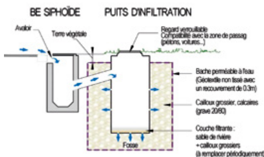
COUPE TYPE D'UN PUIT D'INFILTRATION.
