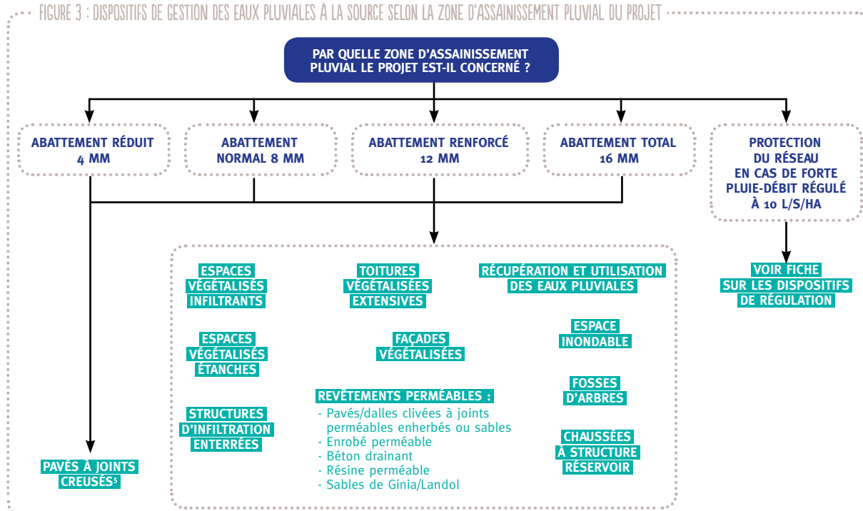
FIGURE 3 : DISPOSITIFS DE GESTION DES EAUX PLUVIALES À LA SOURCE SELON LA ZONE D'ASSAINISSEMENT PLUVIAL DU PROJET
