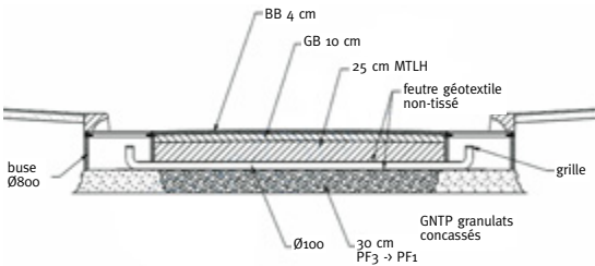
COUPE TYPE D'UNE CHAUSSEE A STRUCTURE RESERVOIR DE TYPE T (FAIBLE TRAFIC) AVEC BOUCHE D'INJECTION.
