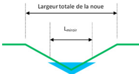
Figure 1 : Illustration de la surface contribuant à l'infiltration pour une noue
