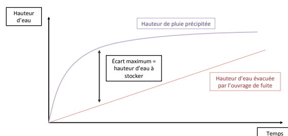
Figure 5 : Illustration de la méthode des pluies
