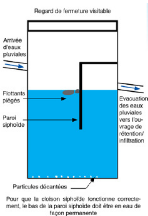
REGARD AVEC DÉCANTATION ET CLOISON SIPHOÏDE La pluie en ville, CG 92
