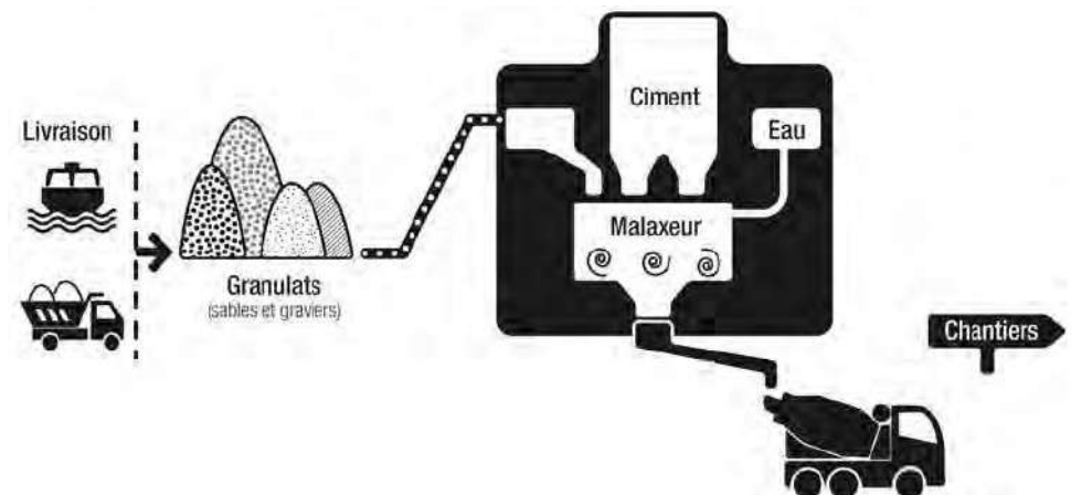
Figure 17 : Schéma explicatif du fonctionnement d'une centrale à béton (source : panorama des granulats en Île-de-France, 2017).
